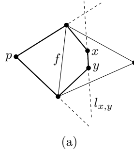
Fig. 13. Observation 13.
