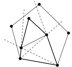
Fig. 7. |H| = 5 .
